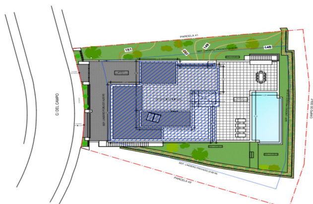
ORDENACIÓN GENERAL DE PARCELA: EMPLAZAMIENTO ACOTADO
